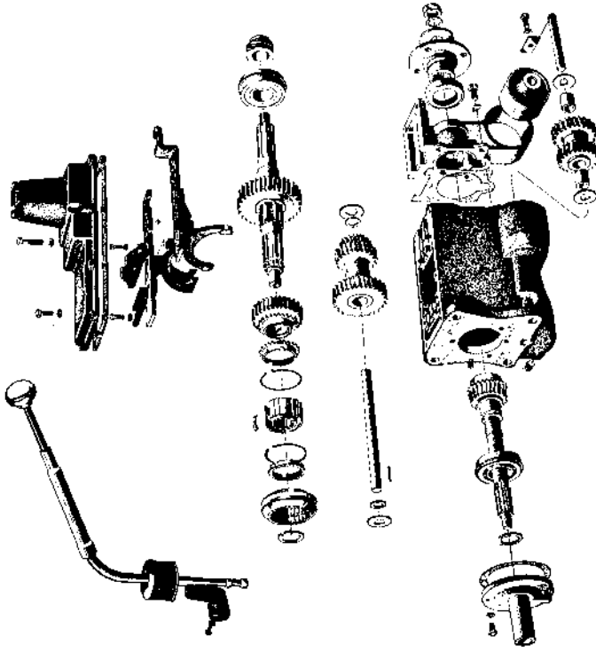
Värelåda.
