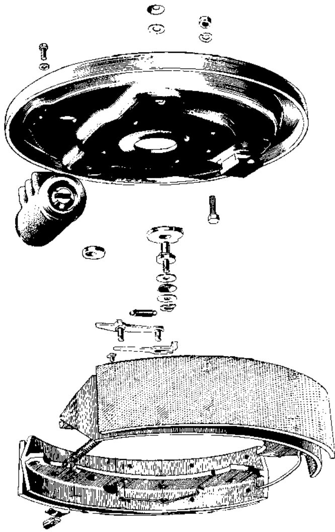
Bromsbackar.
