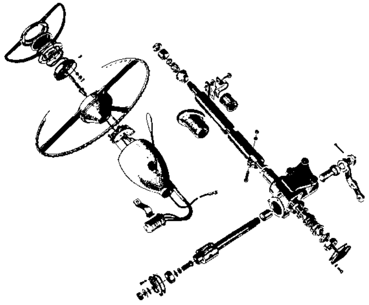
Styrinrätting.
